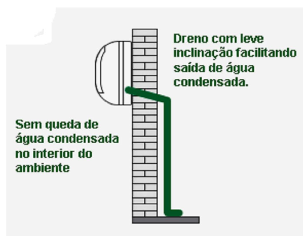
DETALHE Dreno Ar Condicionado sem escala
